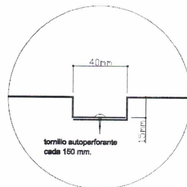
DETALLE BUÑA DE ENCASTRE
